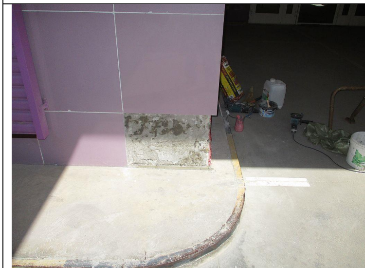
Кор.5, Сек.3, эт.-1 Холодный проезд Ремонт стен -подготовка участка стен -установка плитки
