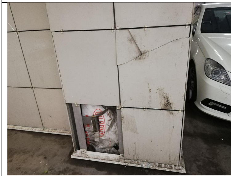
Кор.3, эт.-1 Заглубленный проезд Установка плитки на вентилируемый фасад -установка плитки на вентилируемый фасад
