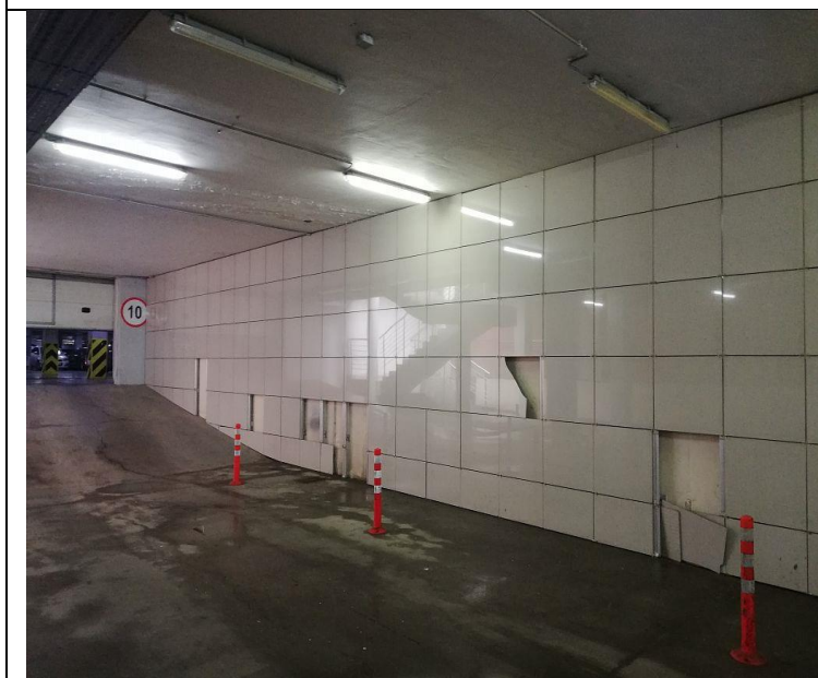
Кор.3, эт.-1 Заглубленный проезд Установка плитки на вентилируемый фасад -установка плитки на вентилируемый фасад
